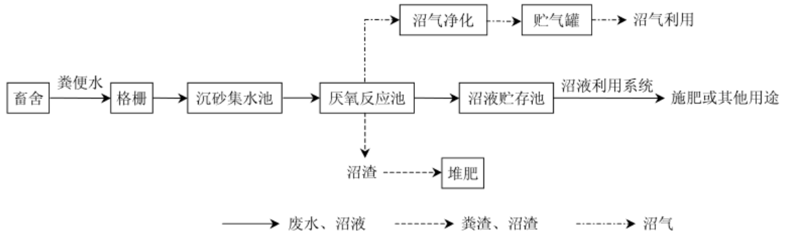
图5.2-2 模式I基本工艺流程
