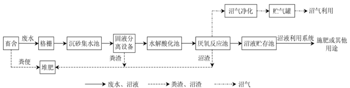
图5.2-3 模式II基本工艺流程
