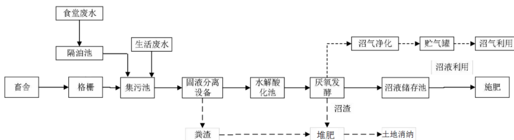
图 5.2-5 项目污水处理工艺流程图
