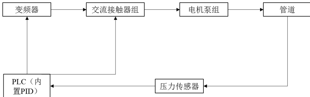
图 6.2-2 恒压供水系统工艺框图
