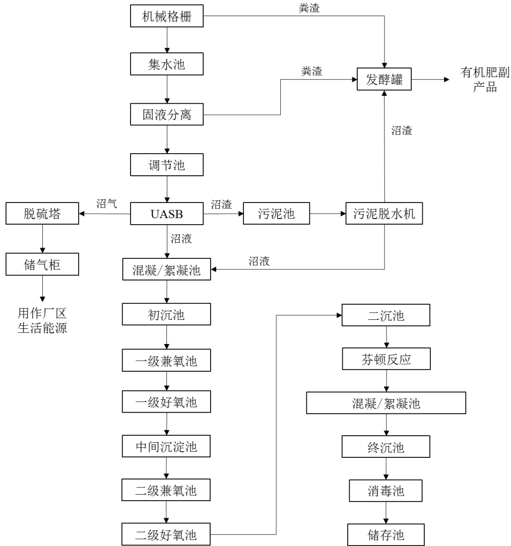
图 6.2-1 项目污水处理工艺流程图
