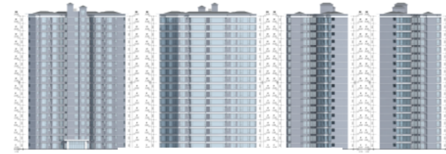
6#、5#楼立面图
