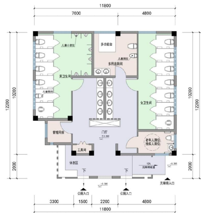
整体式布局公厕平面图
